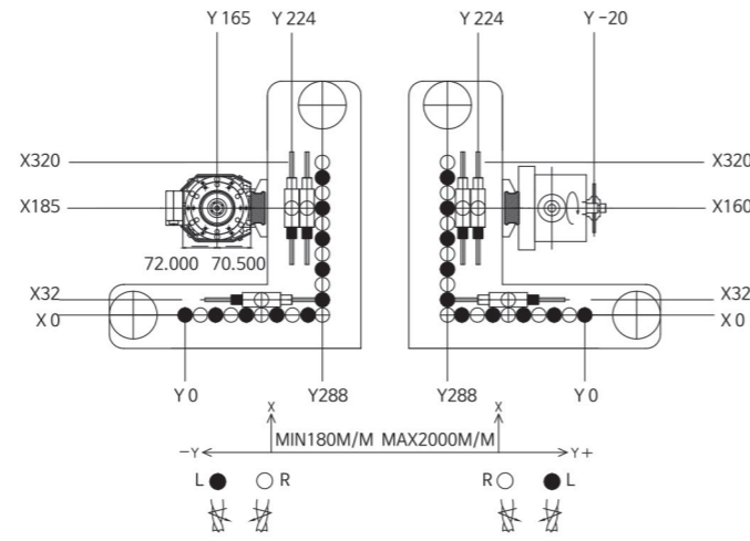
보링헤드 배치도
